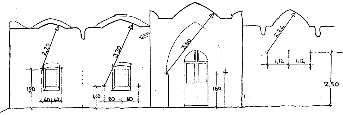
Détails d'acrotère montrant la position des piquets et la longueur des fils de fer.
